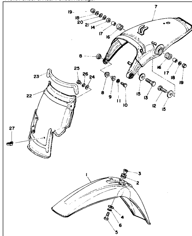
Baugruppe Front Fender & Rear Fender/Kotflügel Figure/Bild 20
