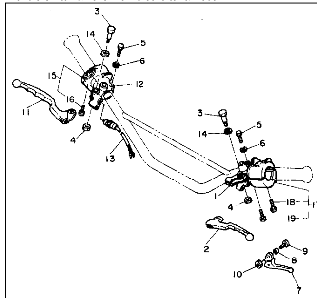
Baugruppe Handle Switch & Lever/Lenkerschalter & Hebel Figure/Bild 37
